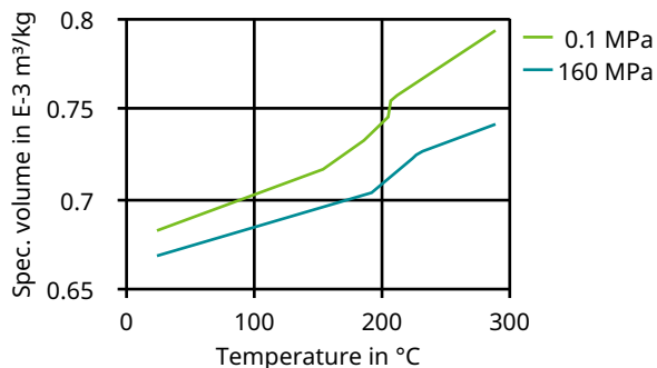
Specific volume-temperature (pvT) (->RADILON A CP400 100 NT)
